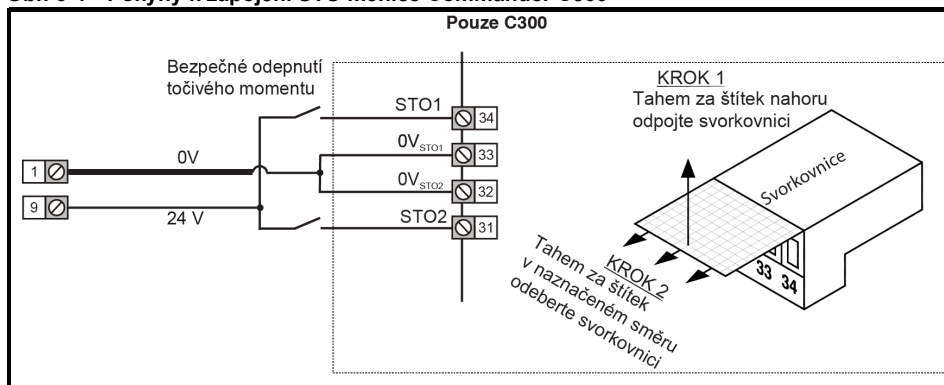
Obr. 6-4 Pokyny k zapojení STO měniče Commander C300
