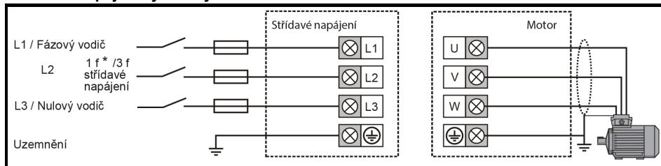
Obr. 6-1 Připojení výkonových svorek
