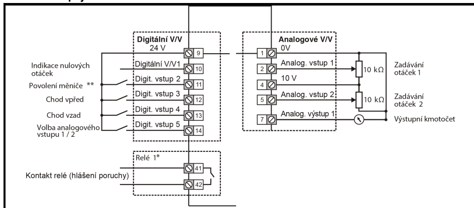
Obr. 6-3 Připojení řídicí svorkovnice měniče Commander C200/C300
