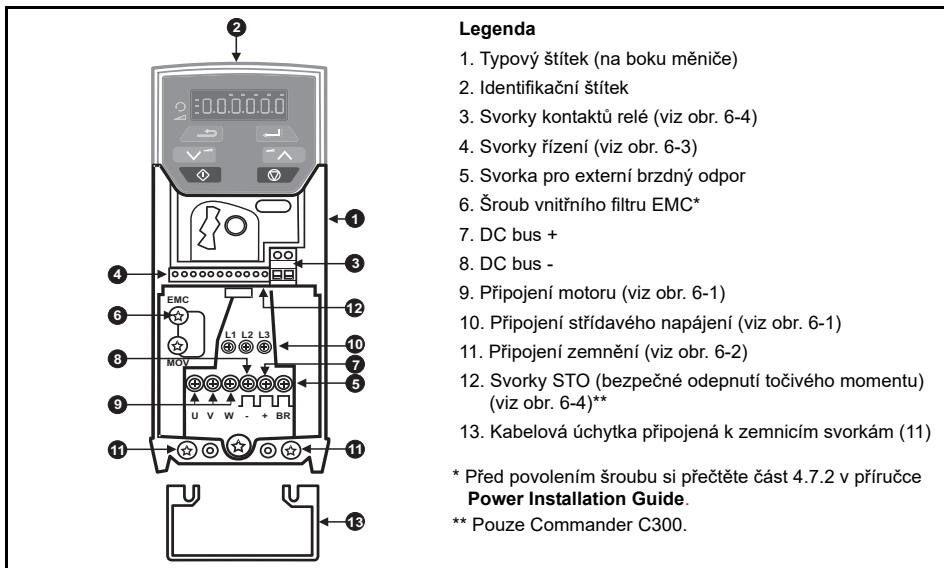
Obr. 1-1 Obrázek měniče s popisem (typová velikost 2)
